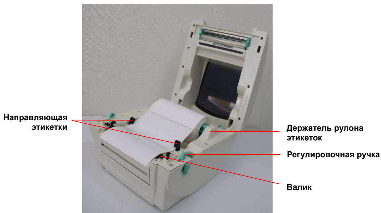
Рис. 7. Установка рулона этикеток (II)
