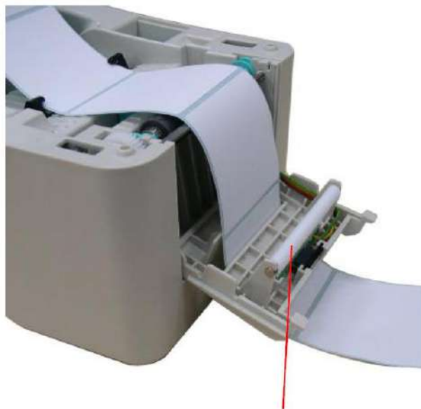
Валик отделителя
